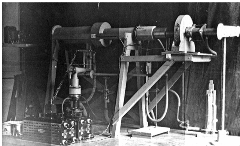
Microscope électronique Trillat Fritz (1931)
