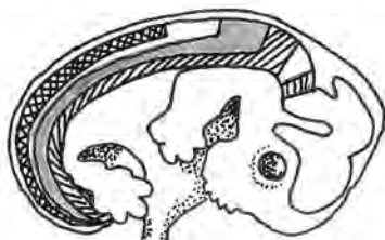
Domaines d'expression de quelques homéogènes chez la Souris
